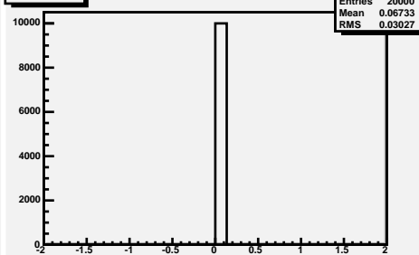
Bottom Pt
