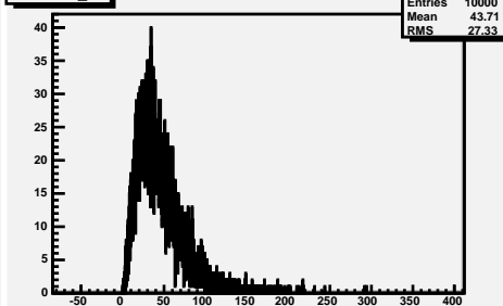
Positron Pt
