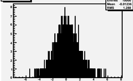
Electron Eta
