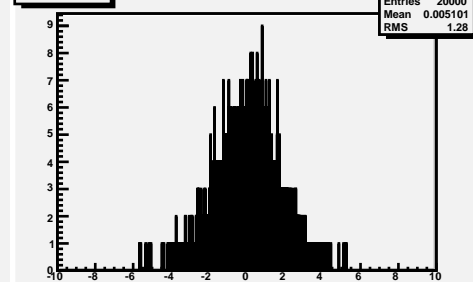
Bottom Eta
