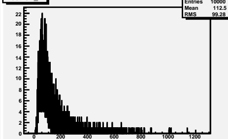
Electron E
