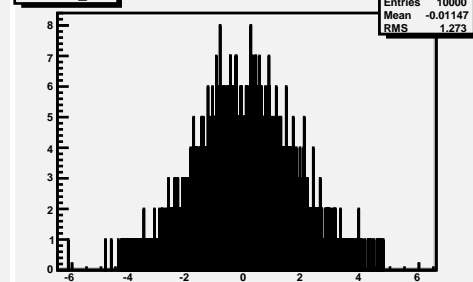
Positron Eta
