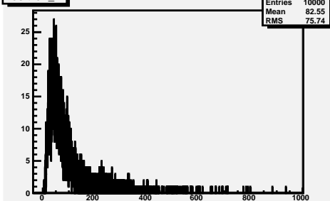
Positron E
