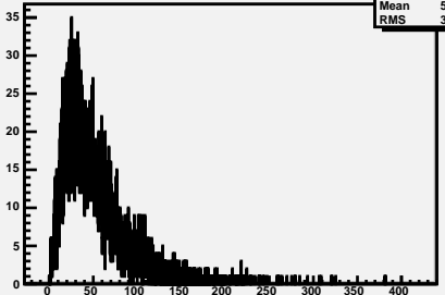
AntiNeutrino_Pt
