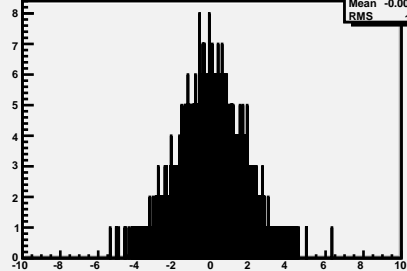
AntiNeutrino_Eta
