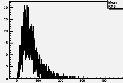
ElectronNeutrino_Pt
